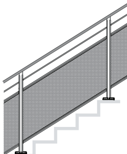
1 lisse intermédiaire
